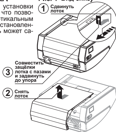
Рис. 4 Вид снизу
