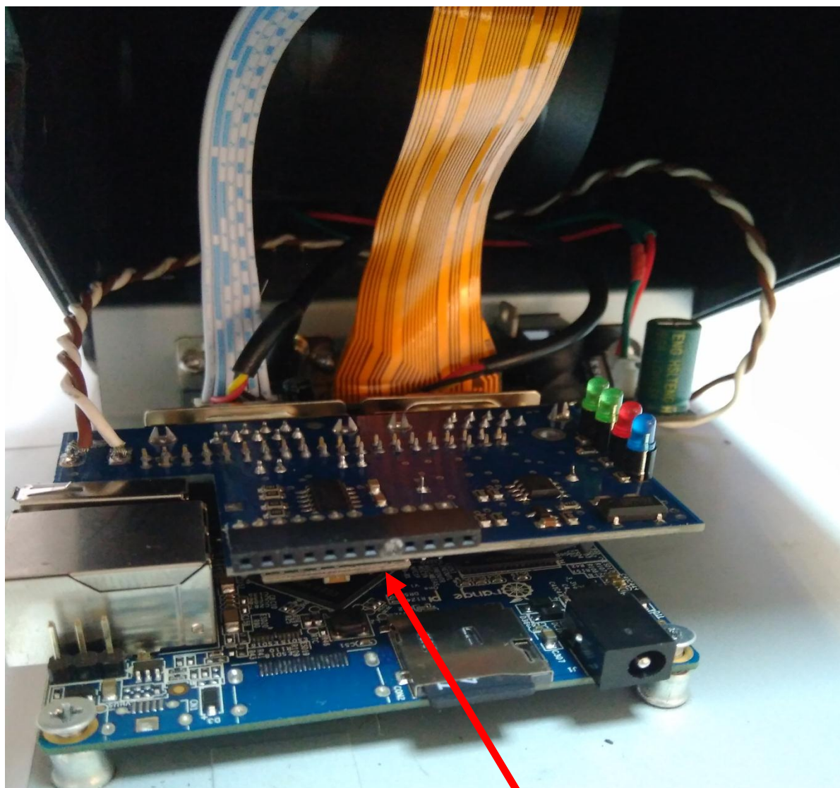
Разъем для подключения ФН
