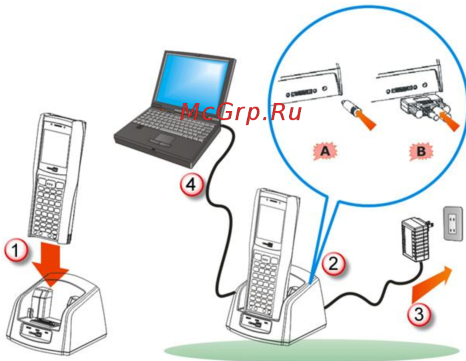
Figure 7: Установка подставки
