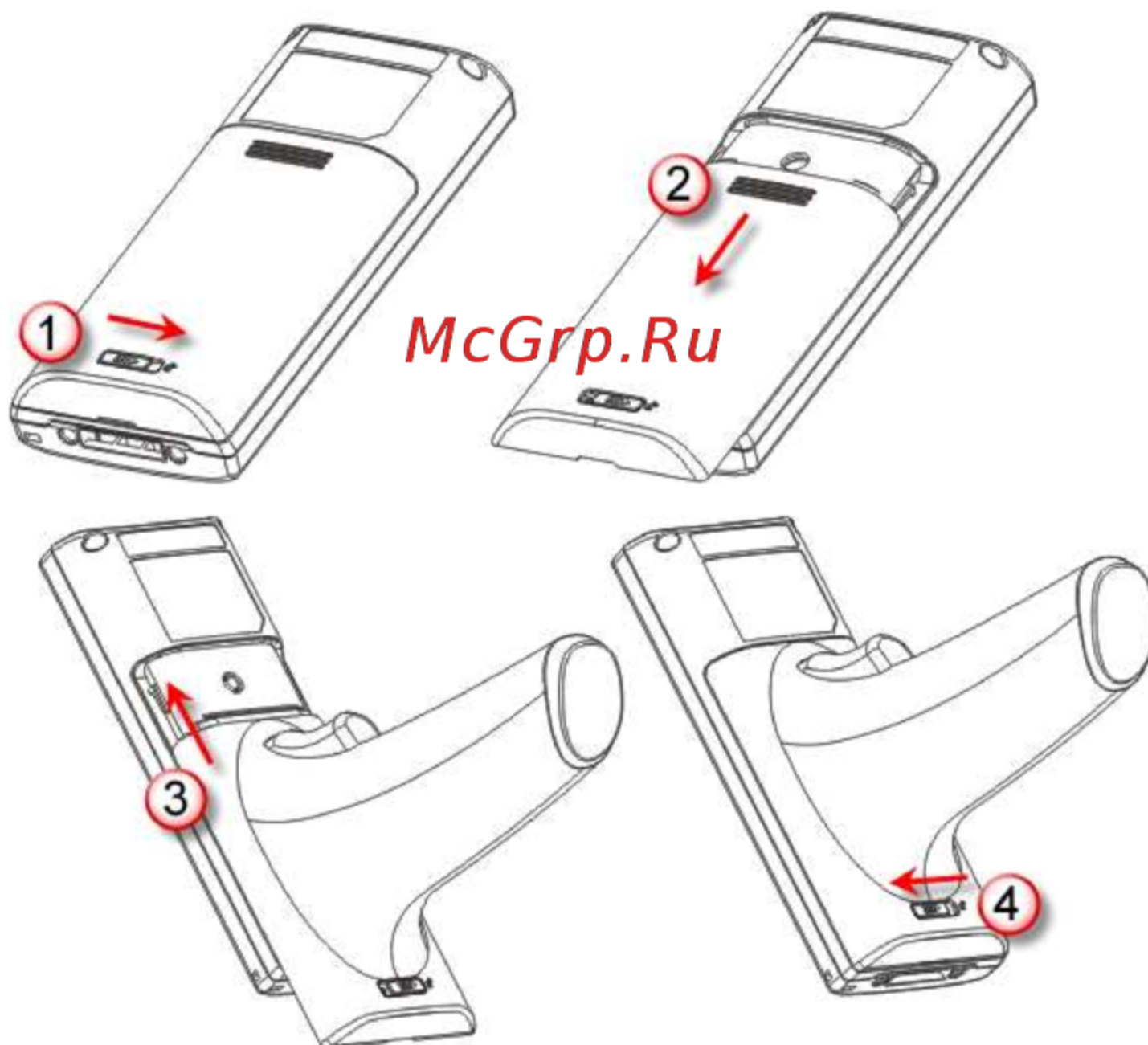
Рисунок 3: Установка пистолетной рукояти
