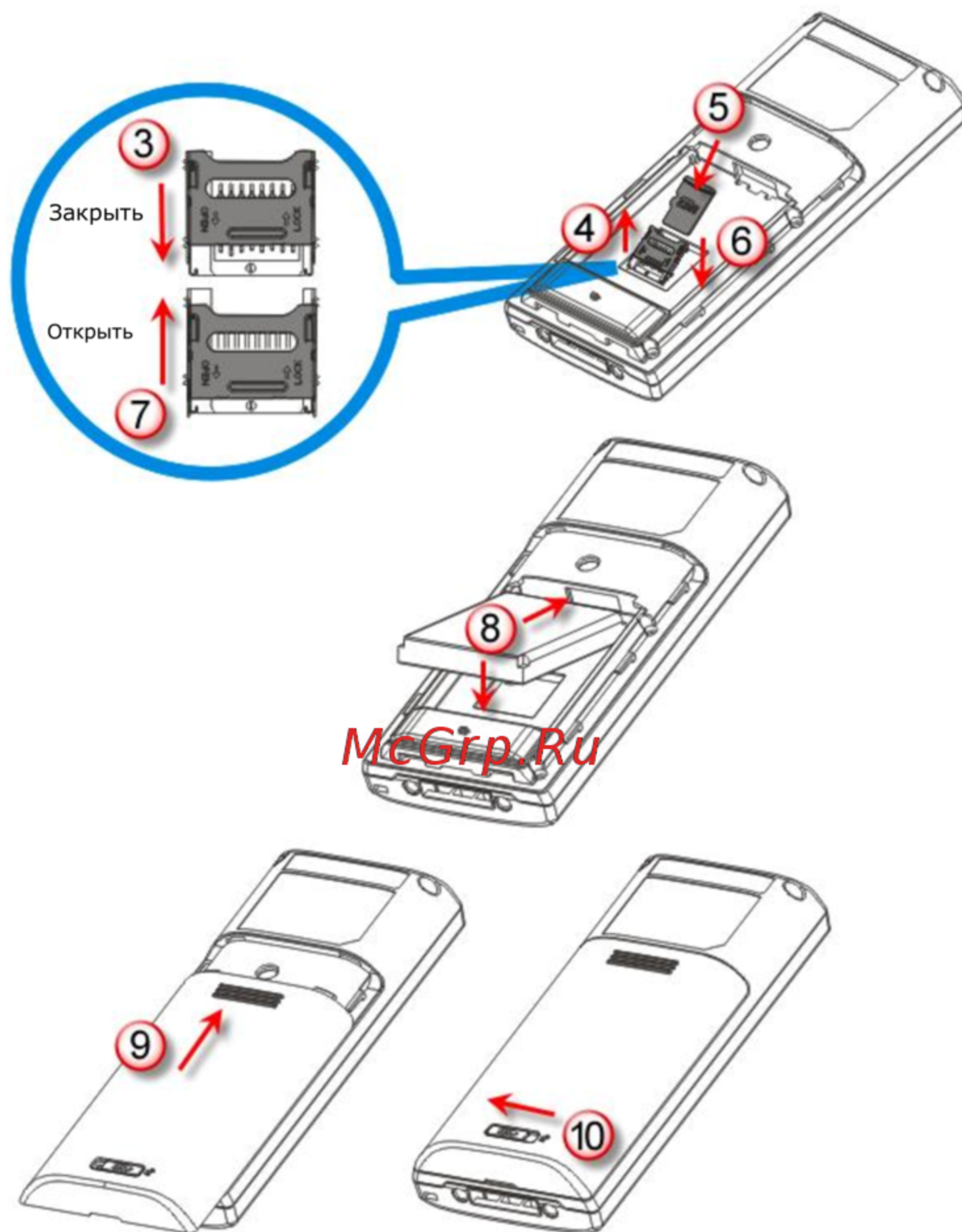
Рисунок 2: Установка основной батареи и flash-карты памяти
