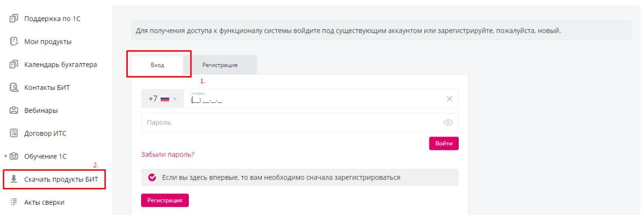
Рисунок 1 - Личный кабинет
