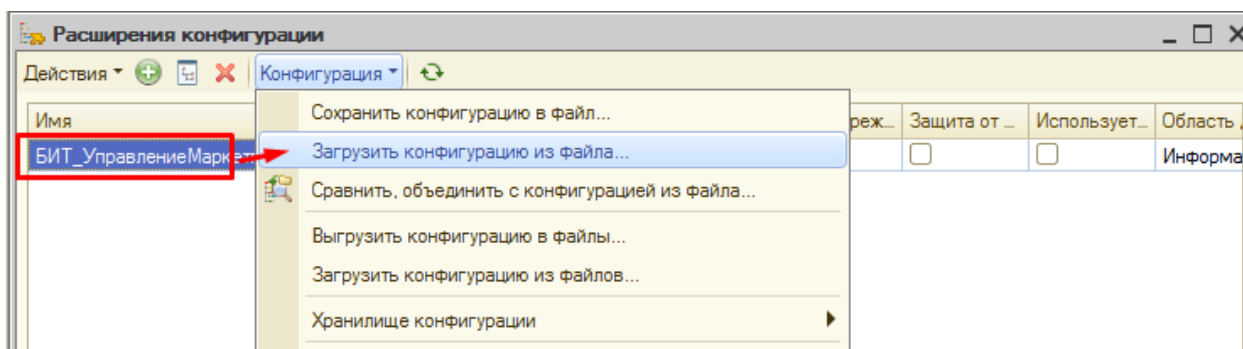
Рисунок 5 - Загрузка конфигурации
