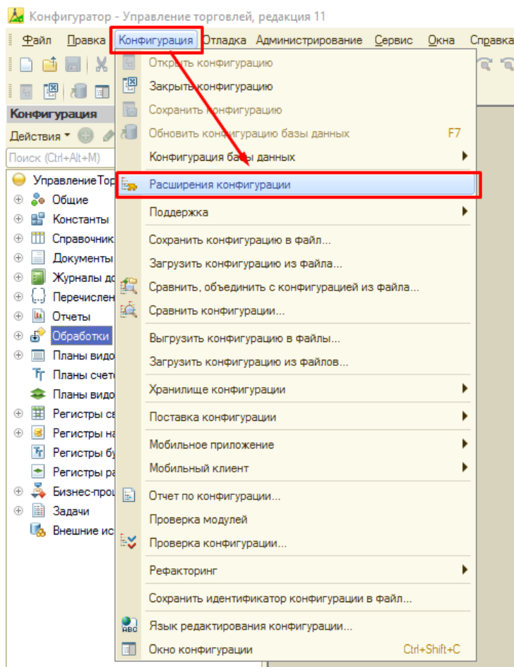
Рисунок 4 - Расширения конфигурации
