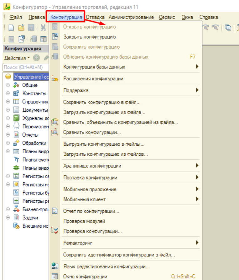
Рисунок 3 - Открытие конфигурации
